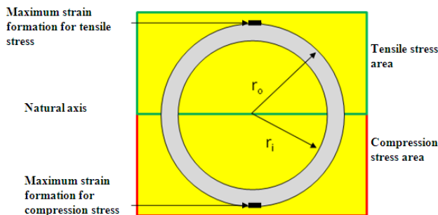
Fig. 4. Pipe dimensions
