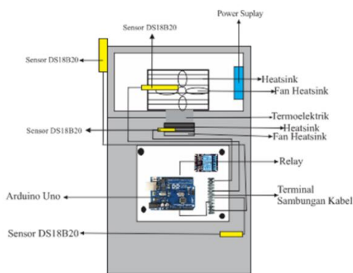
Gambar 6. Mesin penyimpan buah dan sayuran.
