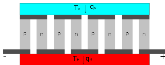
Gambar 1. Sistem Termoelektrik[1].
